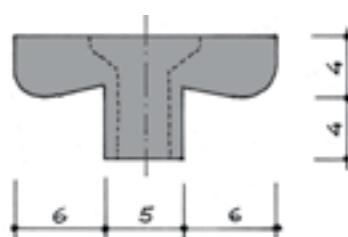
Réf. C535 pour jeu de 5 mm
