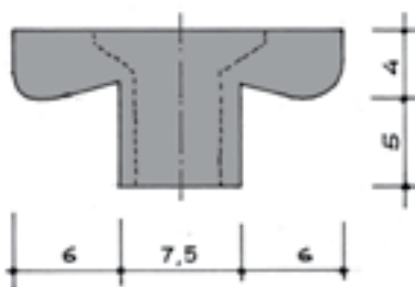
Réf. C755 pour jeu de 7,5 mm
